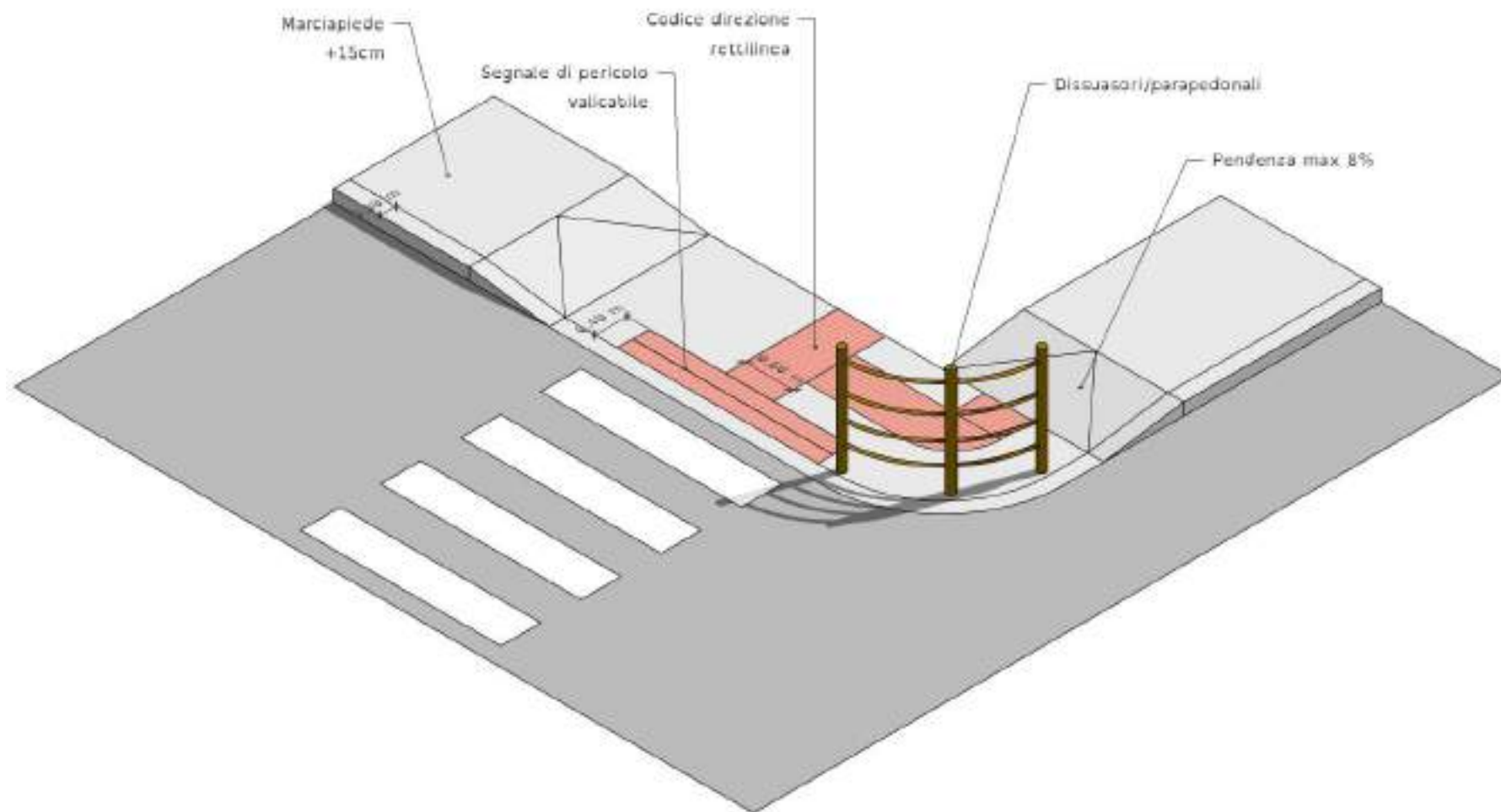
Figura 6-2 Attraversamento pedonale
